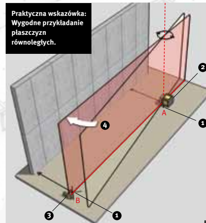
Niwelowanie pionowe: Ze statywu za pomocą zawartego w zakresie dostawy metalowego pałaka lub bezpośrednio na podłożu.
